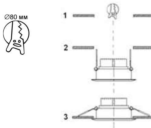
Рис.1. Установка светильника
