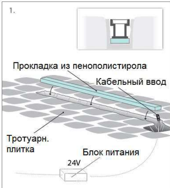
Рис.1-12. Схема монтажа светильника
