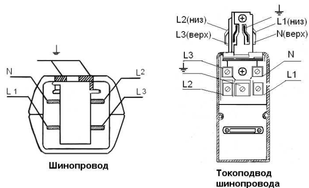
Рис.2. Пример схемы подключения шинопровода 220В.
